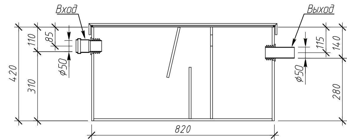
Разрез А-А
